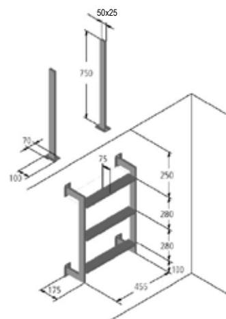
Echelle en inox KLASSIK
