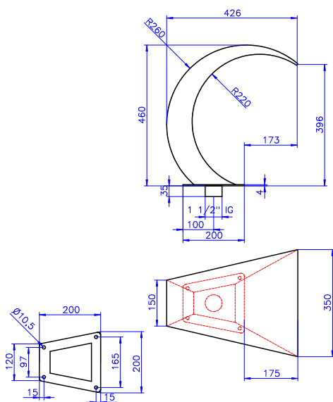
Douche cascade PHOENIX
