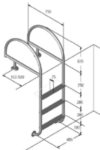
Echelle en inox OMEGA
