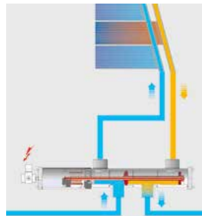
Vanne solaire Besgo
