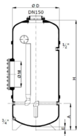
Raccords filetés
