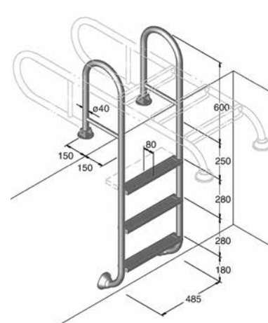
Echelle TINA relevable
