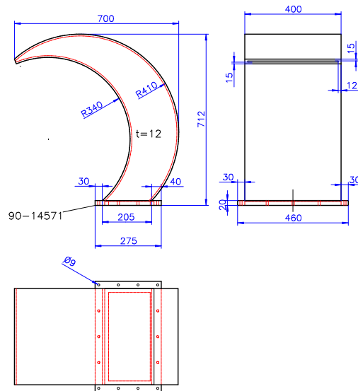
Douche cascade TROPIC
