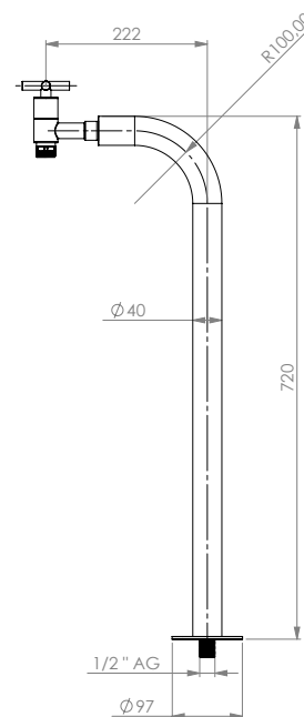
Dispenseur d'eau tube rond
