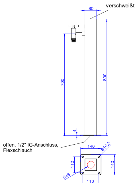
Dispenseur d'eau tube carré
