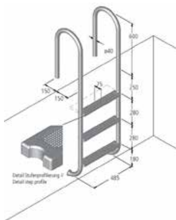
Echelle en inox TINA
